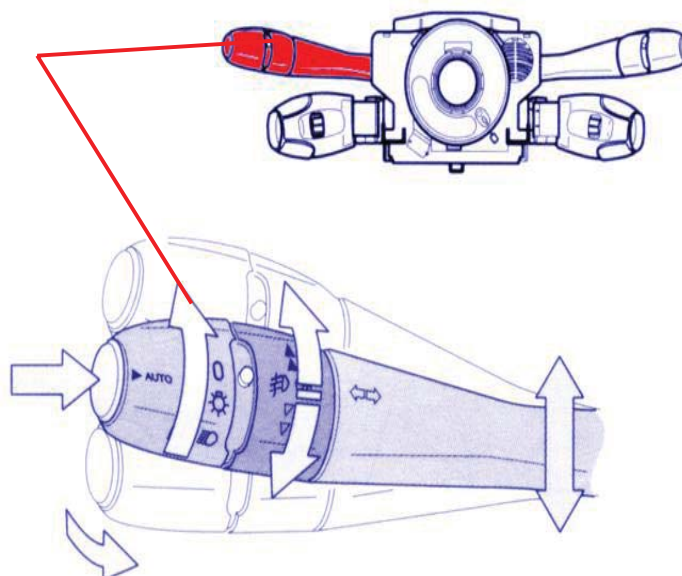
Lighting / Signaling Control Stalk دسته کنترلی نور و روشنایی
